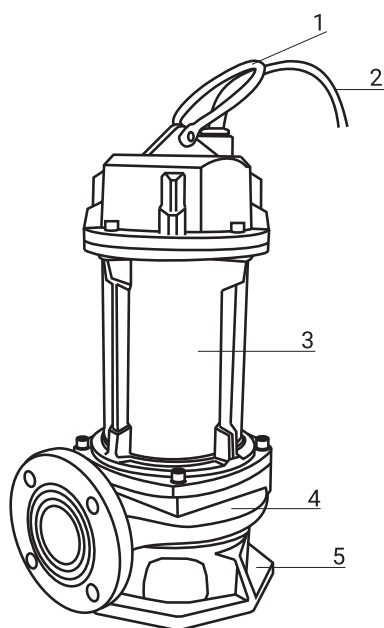
Рис. 2 – Устройство насоса
